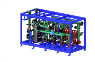
Module : transfert d'énergie Energy Transfer Skid
