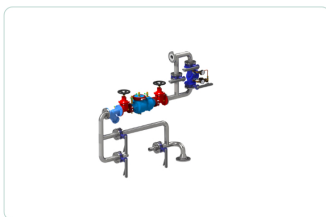
Module : sous-station chauffage / refroidissement District Energy Substation
