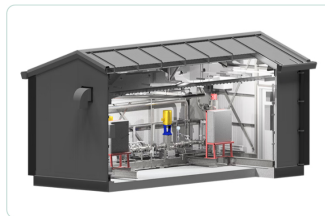
Bâtiment mécanique intégré Full Mechanical Building
